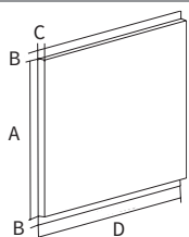
110cm Splashback A: 670mm B: 40mm C: 8mm D: 1102mm
